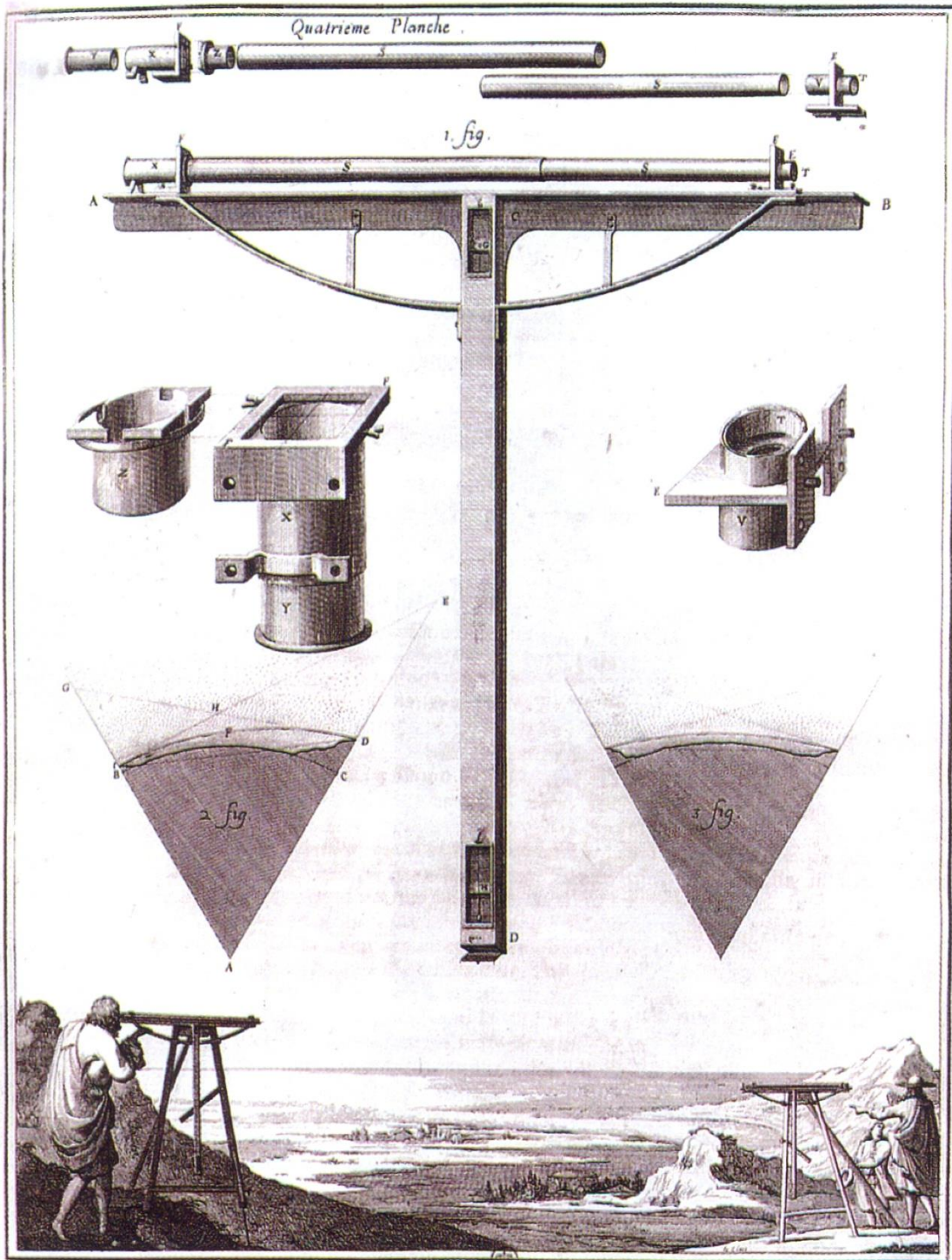
Lunette de nivellement Jean Picard, Traité de nivellement , Paris, 1684.
